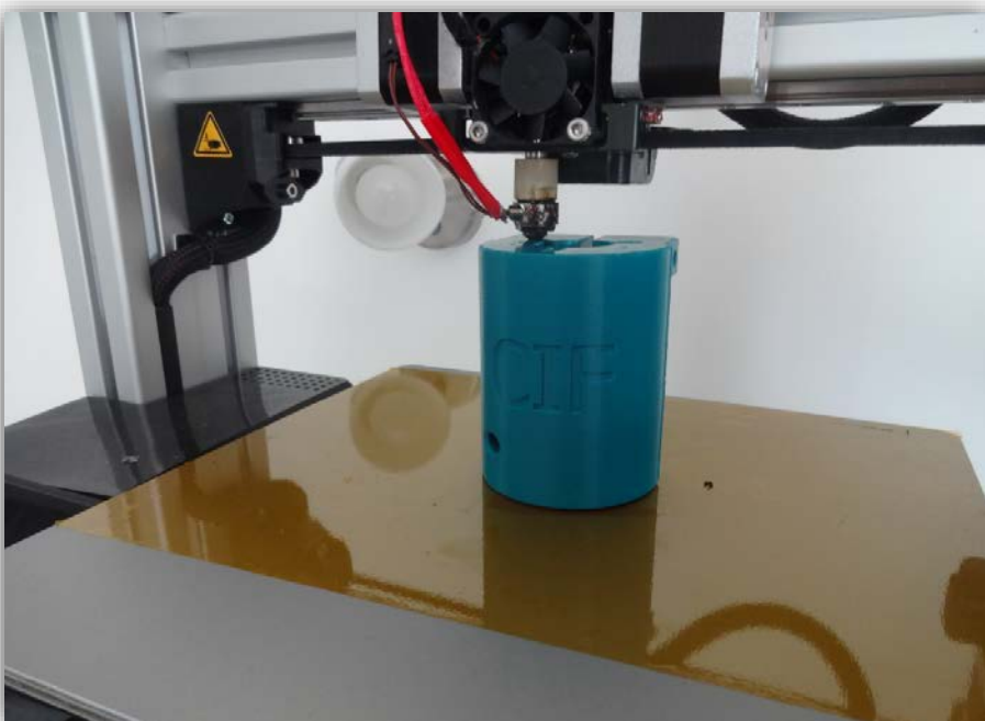
3) Prototype sur imprimante 3D en matière ABS (ou autre)
