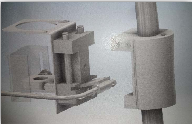
2) Projet sur inventor (fichiers Step, dxf et PDF )
